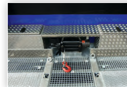
Stirnwandstaukästen mit hydraulischer Seilwinde
