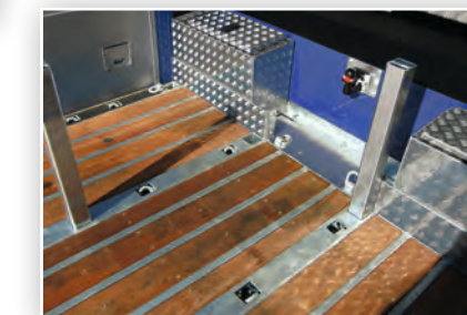
Hartholzboden verlegt in verzinkten Omega-Profilen
