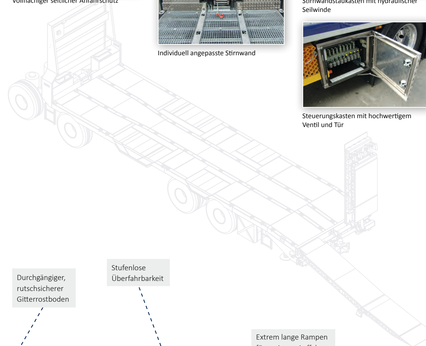
Vollflächiger seitlicher Anfahrerschutz
